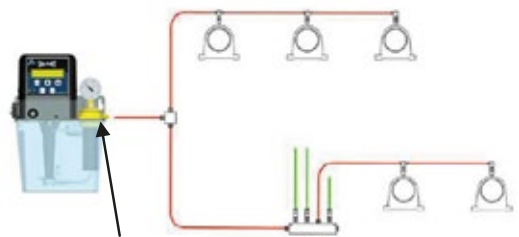
Czujnik ciśnienia
